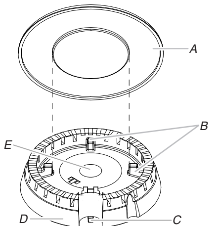
A. Chapeau de brûleur B. Tiges d'alignement C. Allumeur D. Base du brûleur E. Ouverture du tube d'arrivée de gaz
